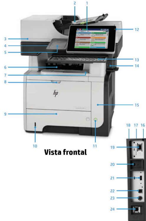
Detalle de los puertos de E/S
